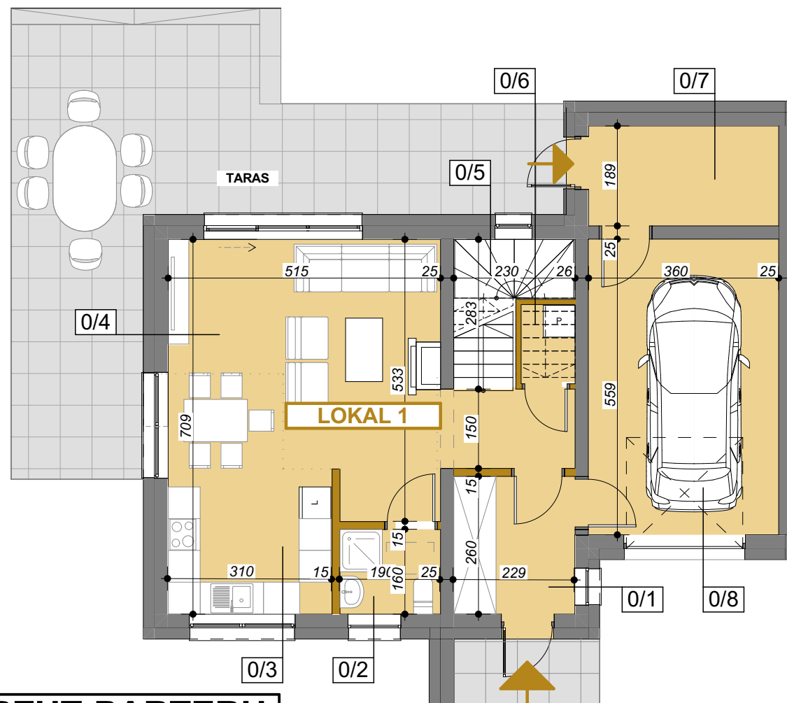
RZUT PARTERU
